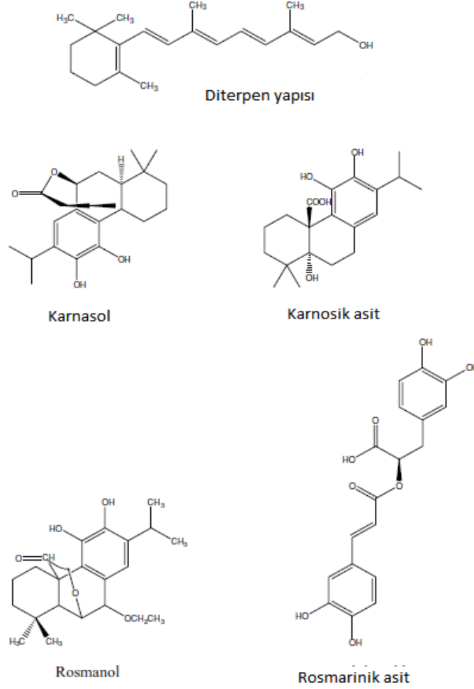
Şekil 16: Bazı fenolik diterpen yapıları
