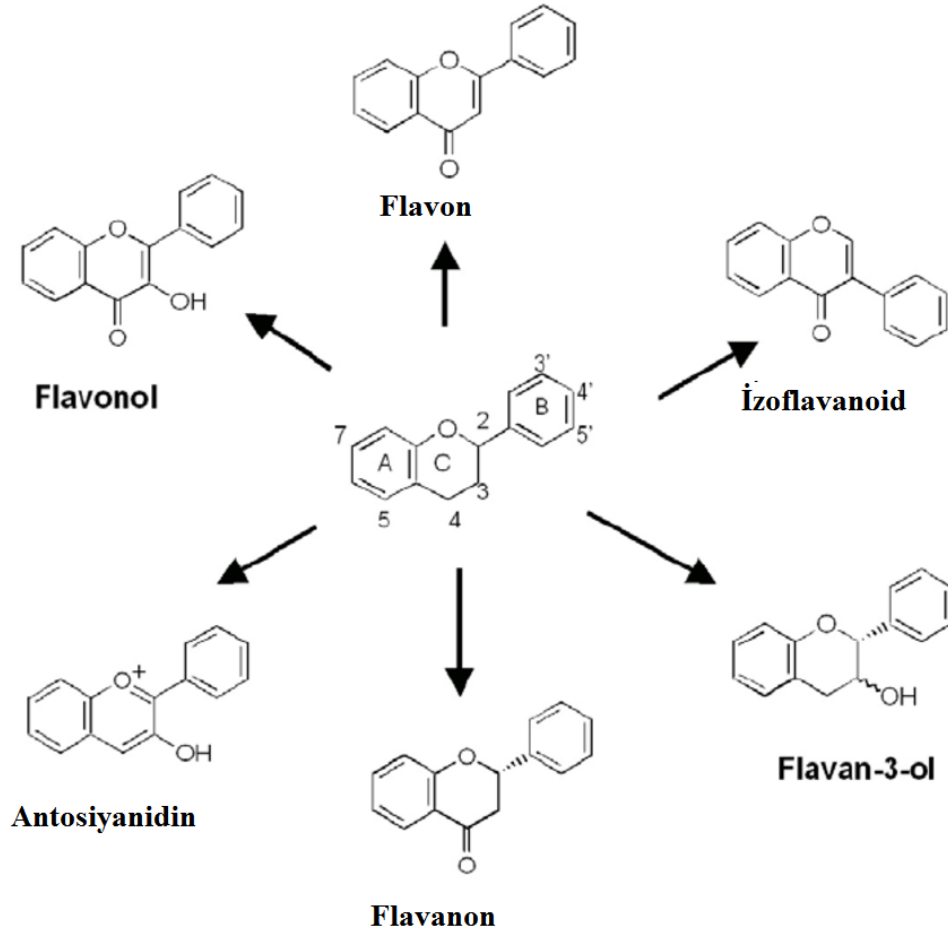
Şekil 19: Temel flavonoid yapıları
