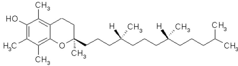
Şekil 14: Tokoferol yapısı
