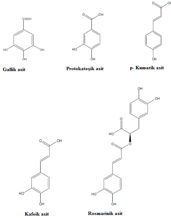
Şekil 18: Bazı fenolik asitlerin yapısı
