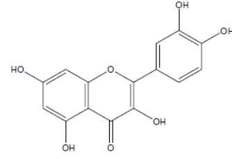
Kuersetin
