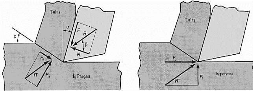
Şekil 2.4: Kesme kuvvetleri şematik gösterimi (Kurşuncu, 2016)
