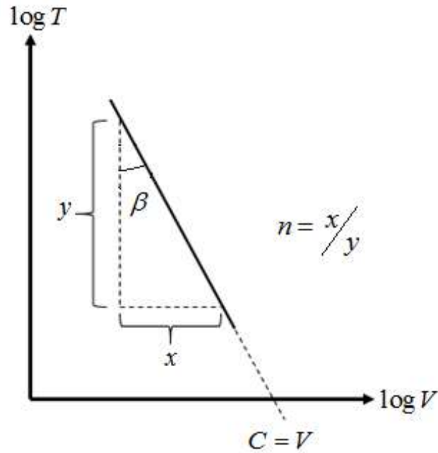
Şekil 2.7: Eğim, n üssü ve C katsayısı (Ay, 2013)
