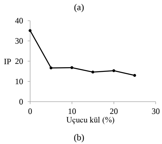
Şekil 5. Farklı kül oranlarına bağlı elde edilen uçucu kül-kil karışımı örneklerinin a) Likit limit (LL) b) Plastisite indisi (IP) değişimi
