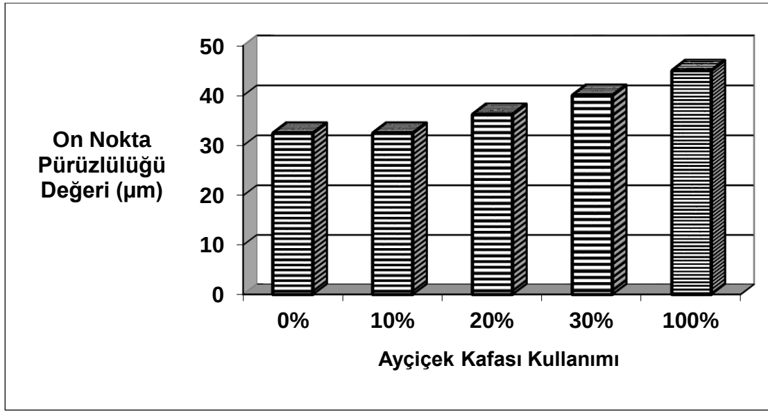
Şekil 8. Ayçiçek tablası kullanımının on nokta pürüzlülüğü değeri üzerine etkisi
