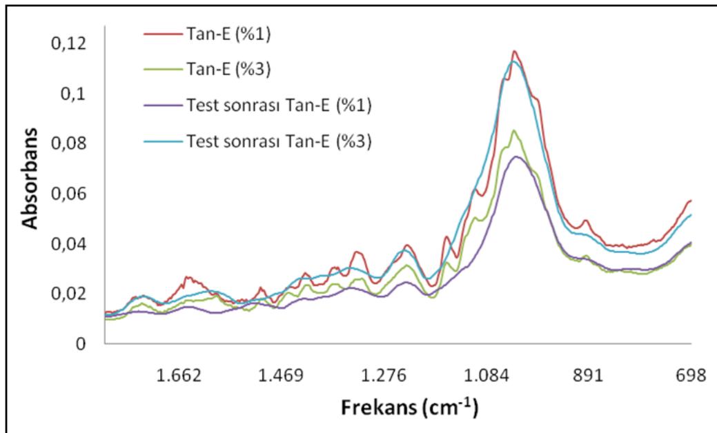
Şekil 5. Mantar çürüklük testi öncesi ve sonrası Tan-E emprenyeli örnekler için FT-IR spektralleri.
