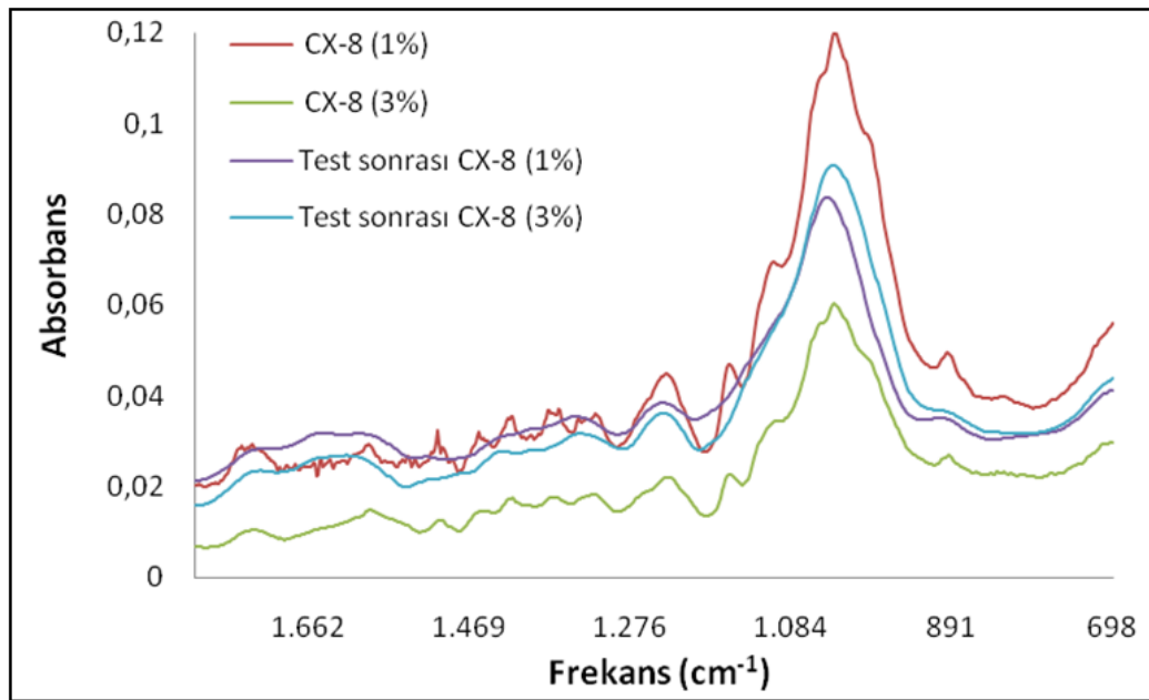
Şekil 6. Mantar çürüklük testi öncesi ve sonrası CX-8 empenyeli örneklerle ait FT-IR spektralari
