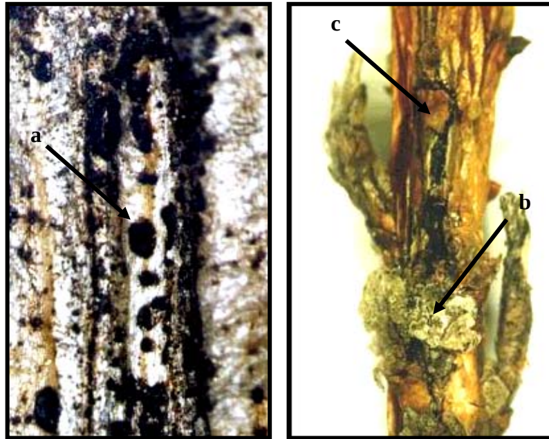
Şekil 1: Melampsora pinitorqua 'nın a) Aecidium b) Reçine c) Kabaran kabuk kısmı ve fungusa ait yapı.
