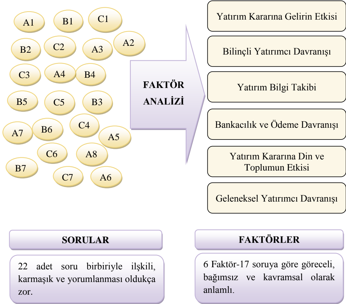
Şekil 4.1: Faktör Analizi Şematik Görünümü
