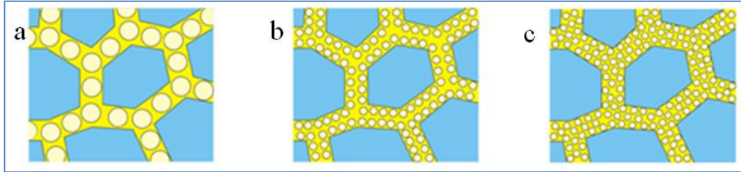
Şekil 36: Simplicolumellate (a), Duplicolumellate (b), Pluricolumellate (c) çizimleri (Punt vd., 2007).
