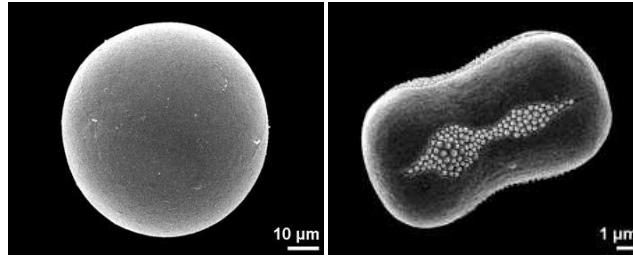
Şekil 30: Psilat SEM görünümü (b) (Hesse vd., 2009).
