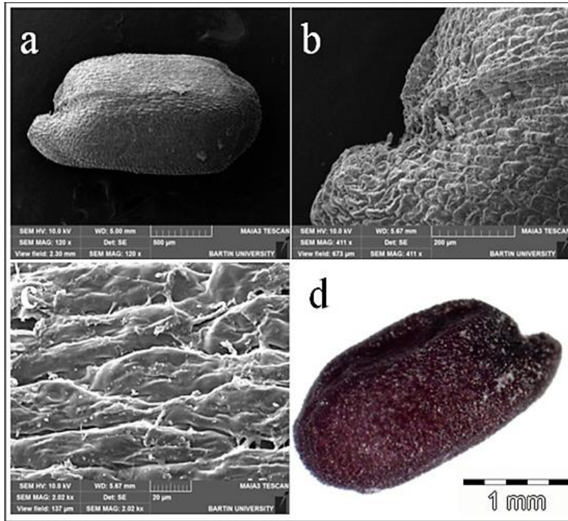
Şekil 66: Acanthophyllum microcephalum tohum SEM genel görünüm (a), tohum SEM hilum görünümü (b), tohum SEM tüberkül görünümü (c), tohum steromikroskop görüntüsü (d).
