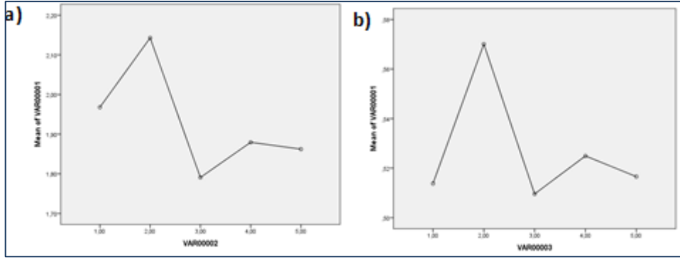
Şekil 71: Ekzin kalınlığı ( F=23,602 , P<0,05 , \text{sig}=0,000 ) (a), intin kalınlığı ( F=4.469, P<0,05 \text{sig}=0,002 ) (b).
