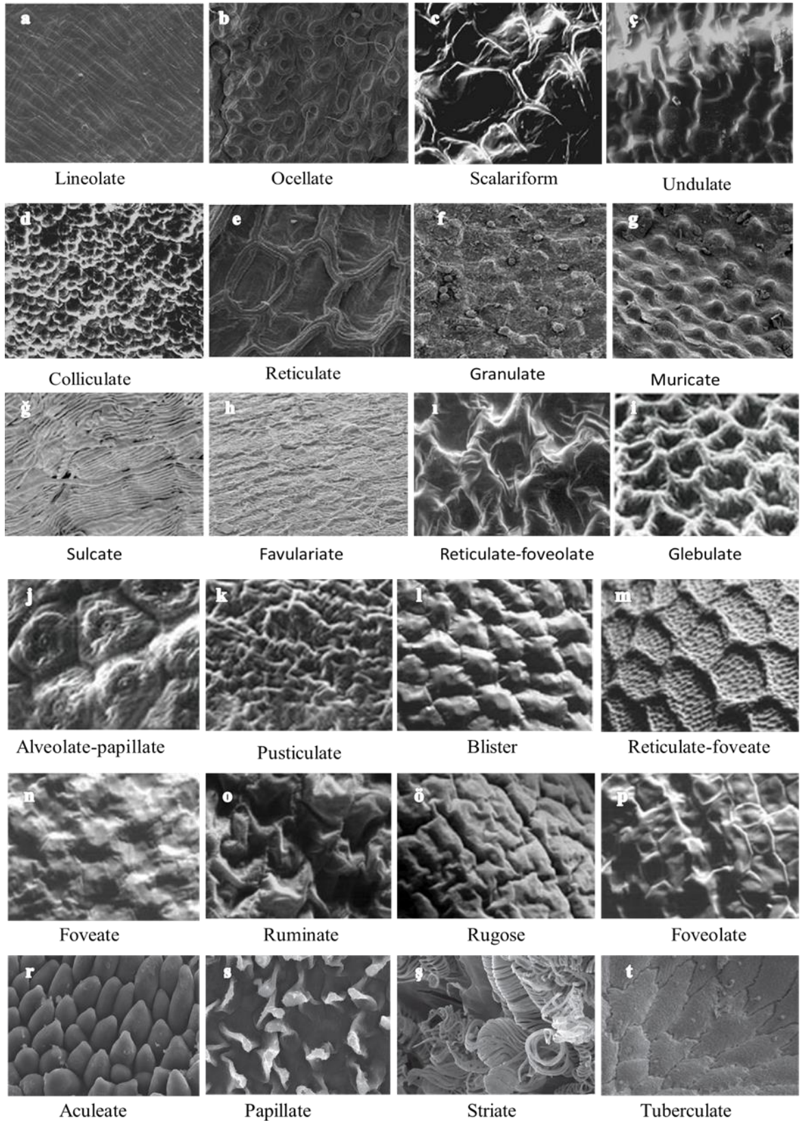
Şekil 52: Tohum yüzey desenleri SEM görünümleri a-e (Moazzeni vd., 2006), f-g (Abid vd., 2014), ğ-h (Abid vd., 2016), ı (Naggar, 2005), i-k (Tantawy vd., 2004), l-p (Zeng vd., 2004), r-ş (Gabr, 2014), t (Arman ve Gholipour, 2013)
