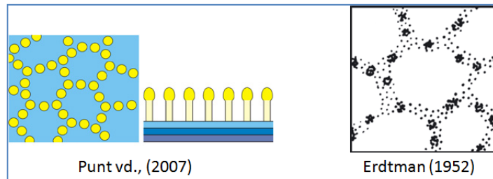
Şekil 37: Retipilate ornamentasyon
