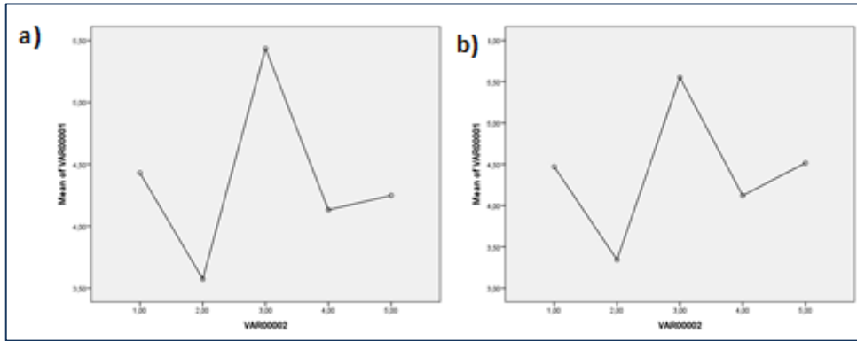
Şekil 72: Por polar eksen uzunluğu grafik gösterimi ( F=13.196, P<0,05 \text{sig}=0,000 ) (a), por ekvatorial eksen uzunluğu grafik gösterimi ( F=17.196, P<0,05 \text{sig}=0,000 ) (b).
