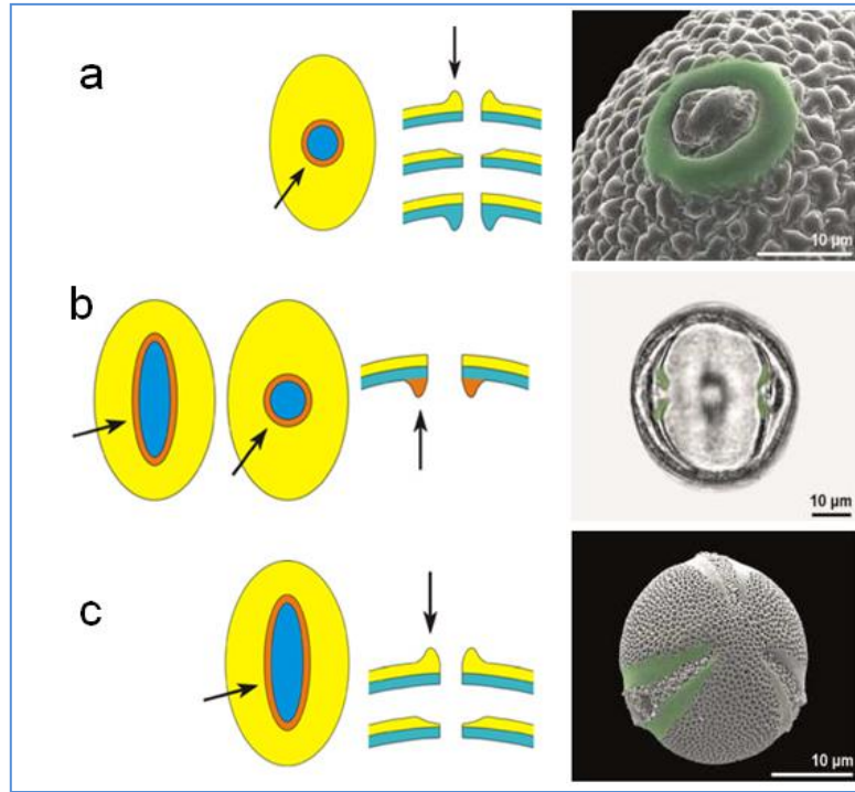
Şekil 18: Annulus (a), Costa (b), Margo (c) (Punt vd., 2007).
